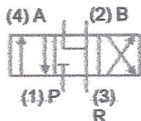
Válvula 4/3 vías, posición central, con conductos de trabajo a escape
