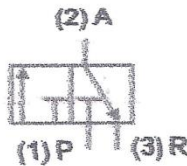
Válvula 3/2 vías Normalmente Abierta
