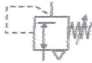
Regulador de presión con agujero de descarga ajustable
