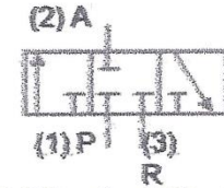
Válvula 3/3 vías, posición central cerrada
