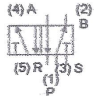
Válvula 5/2 vías
