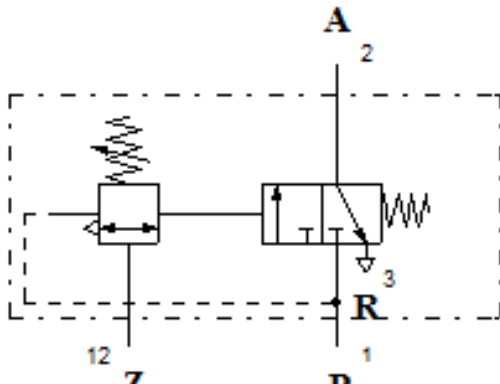
Válvula de secuencia normalmente cerrada
