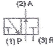
Válvula 3/2 vías Normalmente Cerrada
