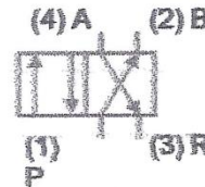
Válvula 4/2 vías
